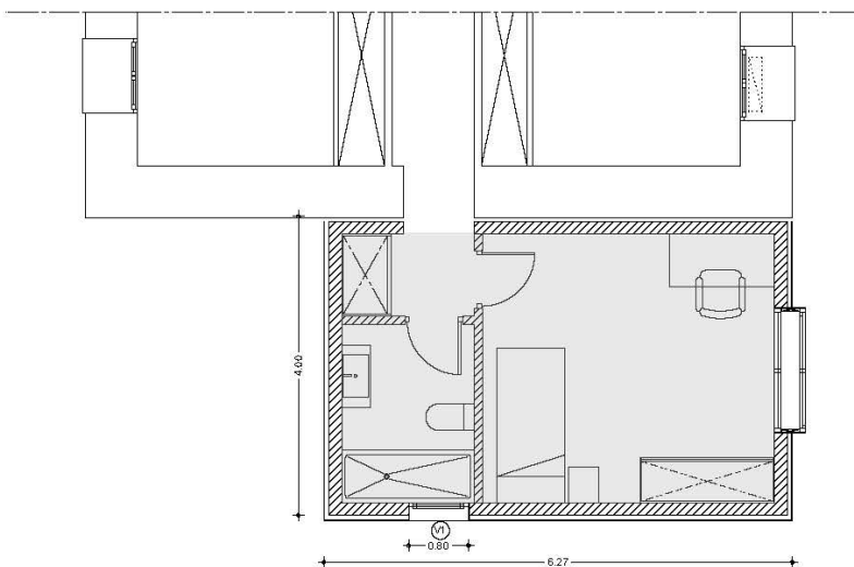
Planta baja.
